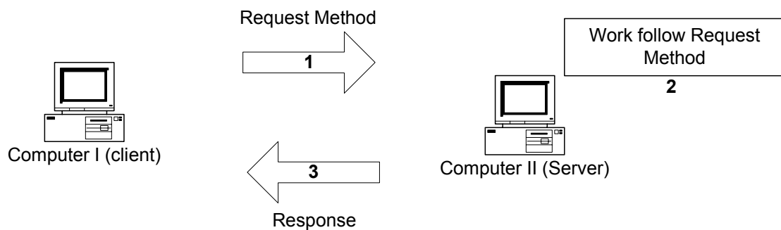
รูปที่ 3-11 แสดงขั้นตอนการเชื่อมต่อในกรณีที่เครื่องไคลเอนต์เป็นเครื่องคอมพิวเตอร์ส่วนบุคคล
