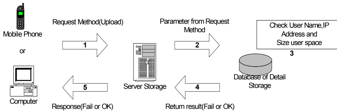
รูปที่ 3-10 แสดงขั้นตอนการเชื่อมต่อระหว่างเครื่องไคลเอนต์กับเซิร์ฟเวอร์ที่ให้บริการพื้นที่ในการสำรองข้อมูล
